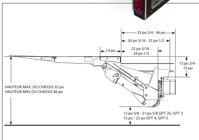
Dimensions du hayon élévateur et exigences de montage du GPT
